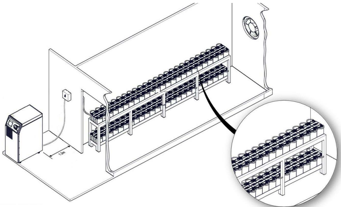
Размещение внешних АКБ на стеллажах
